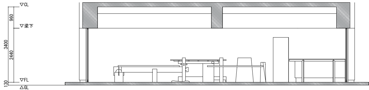
断面図
